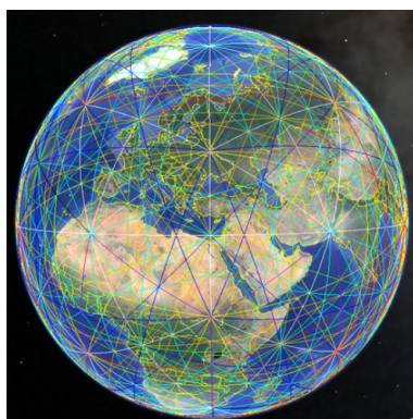
Griglia magnetica terrestre secondo dati biologici
